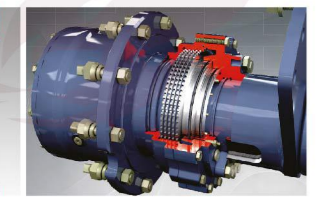
Ведущий мост с тормозами мокрого типа
